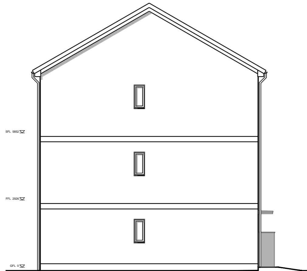
SIDE ELEVATION 1 OP 1 - 30° roof
